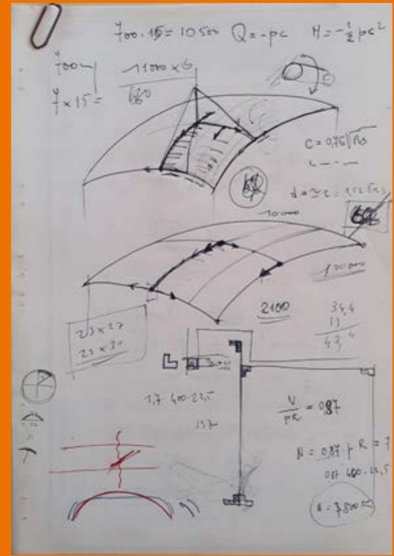
Calcoli per la copertura della piazza centrale ortofrutticola di Trento, [1961] Foto Fabio Campolongo (2020) APTn, AEA, fald. 2, fasc. 135
