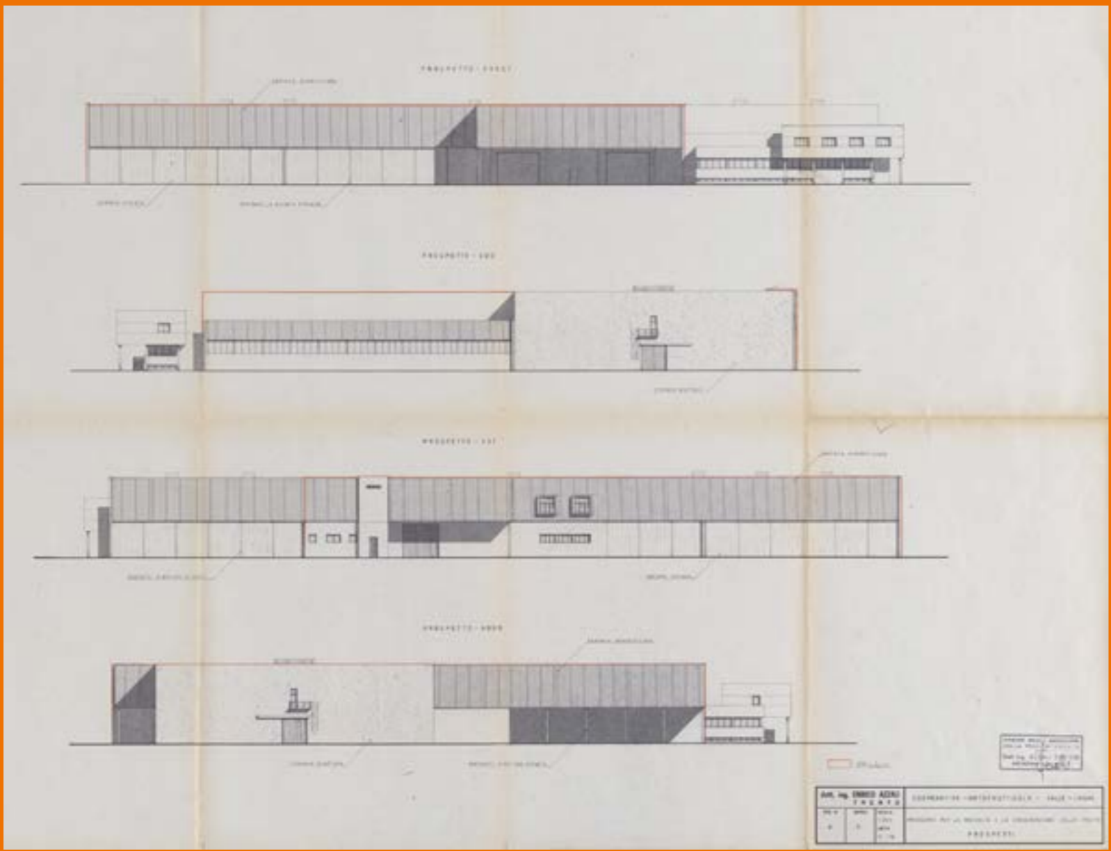
Magazzino per la lavorazione e la conservazione della frutta, per la Cooperativa Ortofrutticola Valle dei Laghi, Pietramurata, prospetti e pianta [1970 ca.] APTn, AEA, b. 51
