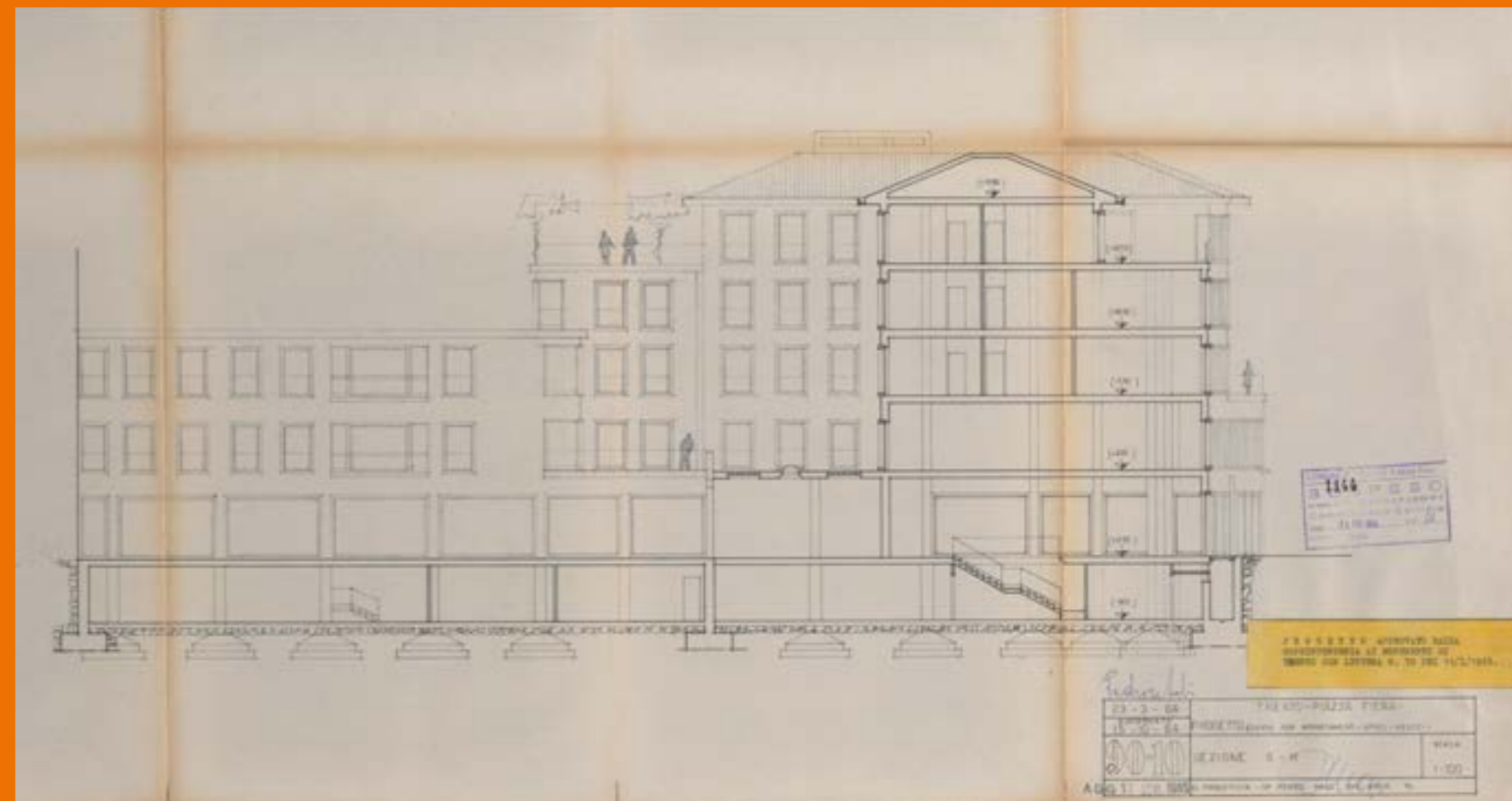
Progetto di edificio per uffici, appartamenti e negozi, piazza della Fiera, Trento. Schizzo prospettico, 1964, e sezione, 11 gennaio 1965 APTn, ARM, sc. 39, b. 90
