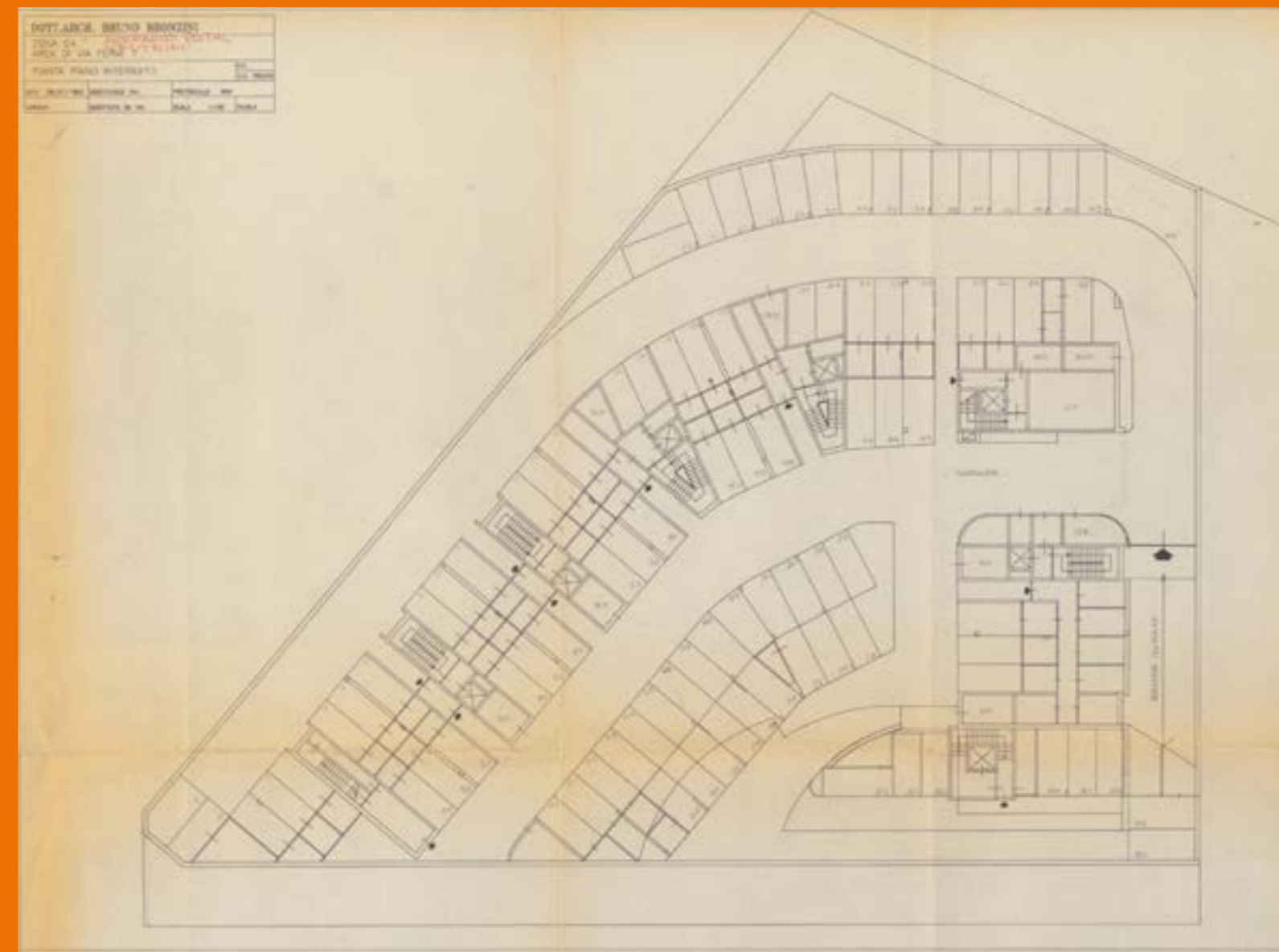
Progetto "via Fermi 1993" (case ITEA), Trento, in collaborazione con Bruno Bronzini e Piera Ventrini. Pianta piano interrato APTn, AACP, sc. 16, cartella 1992-1993
